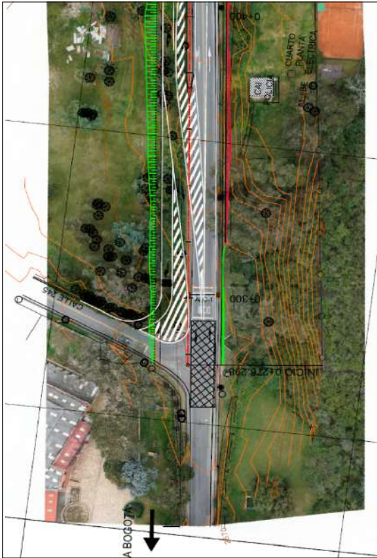
Diseño en planta de la intersección carrera Séptima - Calle 245
