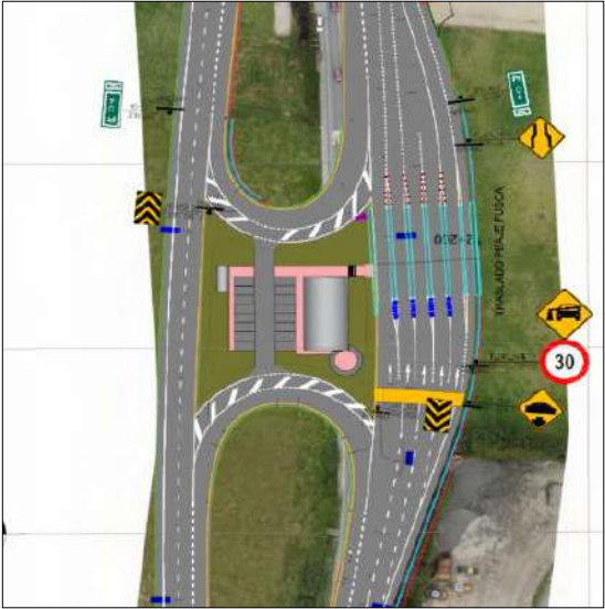
Detalle del Peaje proyectado
