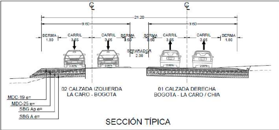
Sección transversal típica de la doble calzada en la UF-1
