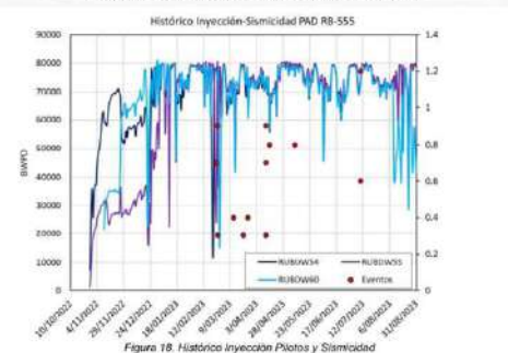
Figura 18. Histórico Inyección Pilotos y Sísmicidad
