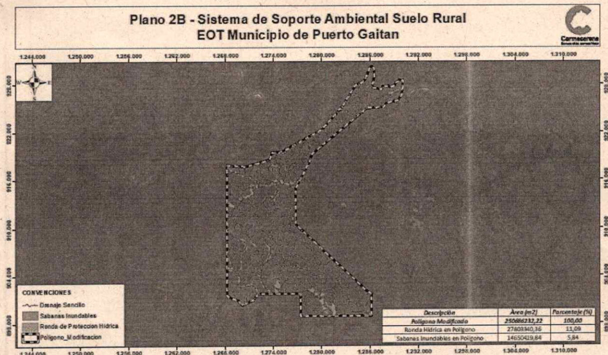
Figura 2. Identificación de ecosistemas estratégicos.
