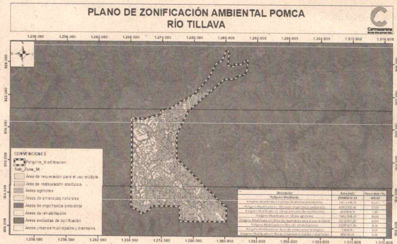
Figura 1. Plano de zonificación Ambiental POMCA Río Tillavá
