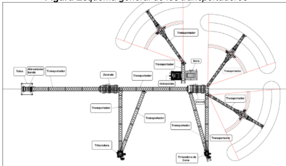
Figura Esquema general de los transportadores
