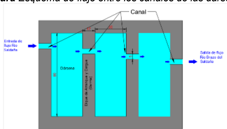
Figura Esquema de flujo entre los canales de las dársenas.
