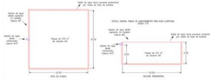
Figura Esquema general del tanque de almacenamiento de agua
