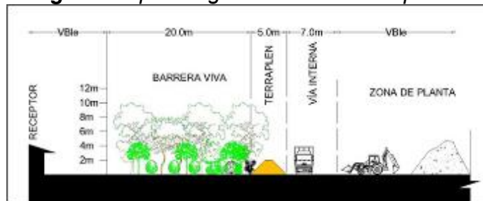
Figura Esquema general de los terraplenes
