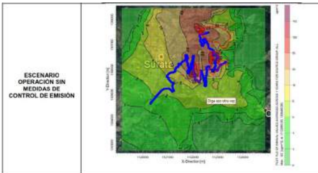
Figura 4-12. Isoplethas PM 10 Anual Sector Padilla
