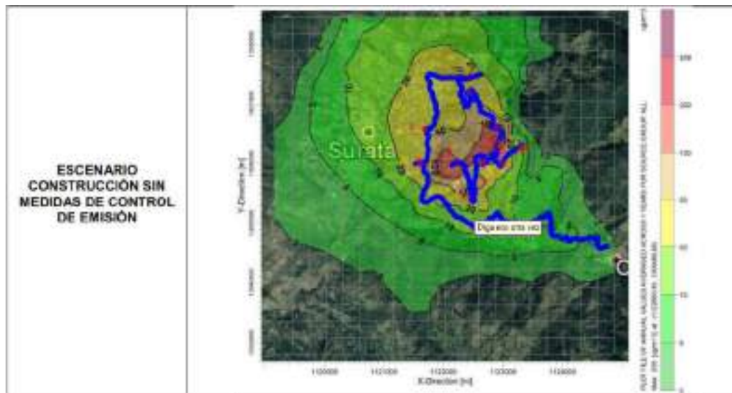
Figura 4-11. Isoplethas PM 10 Anual Sector Padilla
