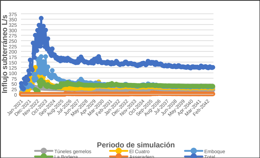
Figura Error! No text of specified style in document. -1 Estimado de influjos subterráneos en la mina y los túneles gemelos Fuente: Información adicional del EIA para solicitud de Licencia Ambiental del “Proyecto de Explotación Subterránea de Minerales Auroargentíferos Soto Norte”. Presentada mediante 2020003948-1-000 del 13/01/2020 (VITAL 3500090006326220002). SOCIEDAD MINERA DE SANTANDER S.A.S.
