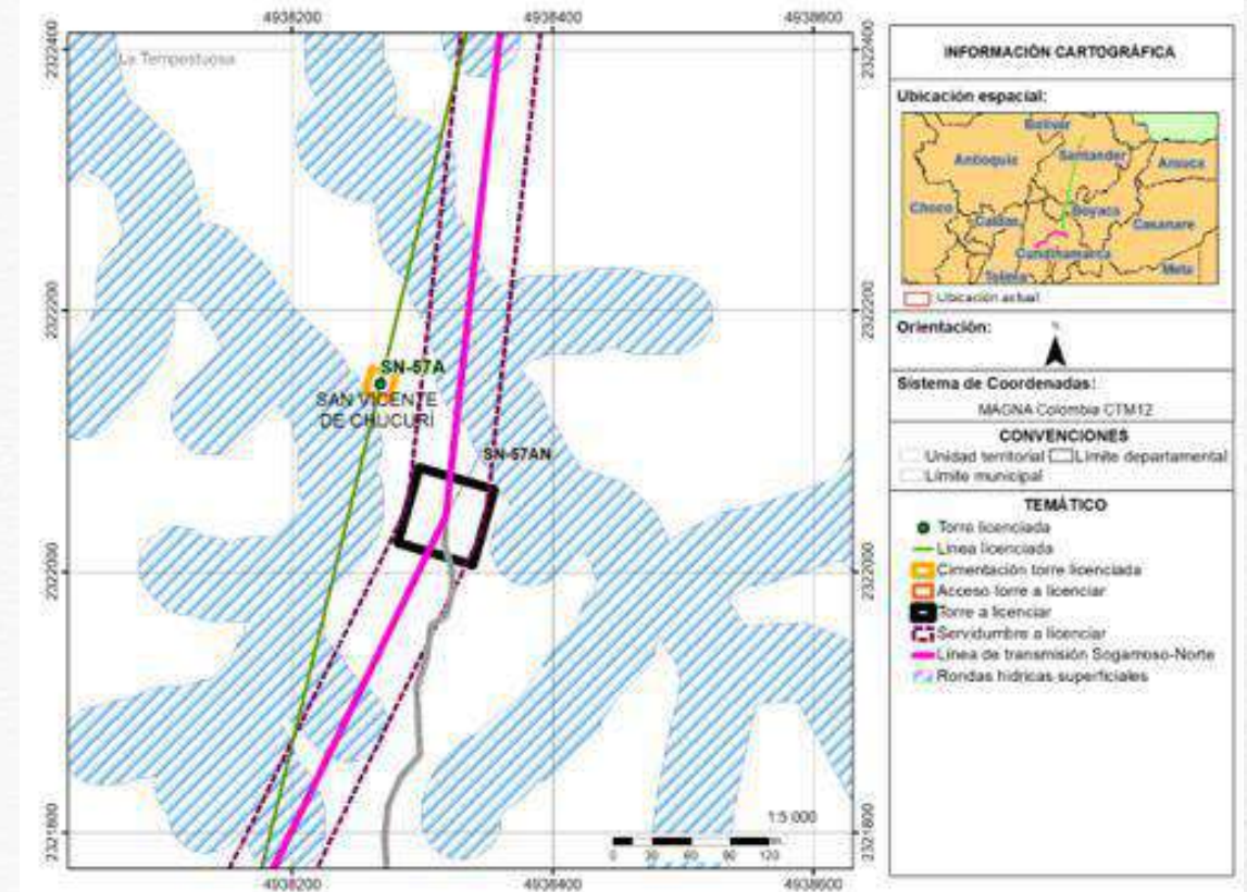
Figura 3-8 Reubicación de la torre SN 57AN
