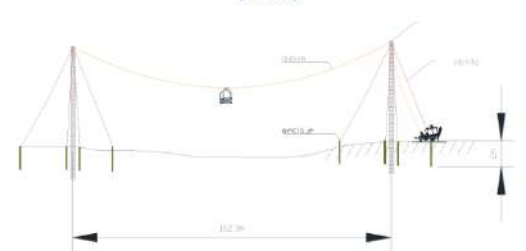
Figura 10-6 Diseño y estructura del sistema de transporte con teleférico y canasta (Tarabita)
