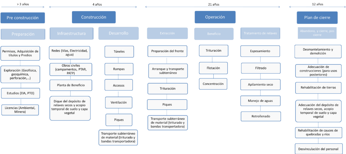
Figura.3 Flujo diagrama de las fases del Proyecto Soto Norte. Fuente: Sociedad Minera de Santander, 2018.
