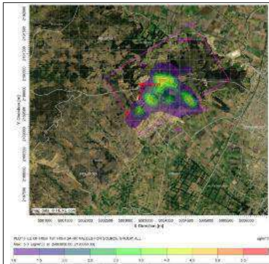
Mapa de dispersión PM2.5 a 24 horas
