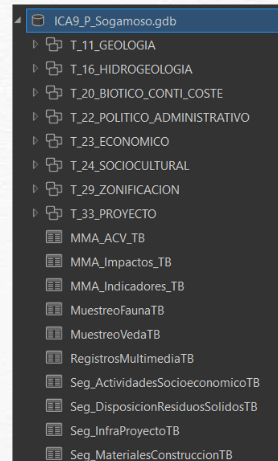
Captura de pantalla de la estructura del MAG “ICA9_P_Sogamoso.gdb”
