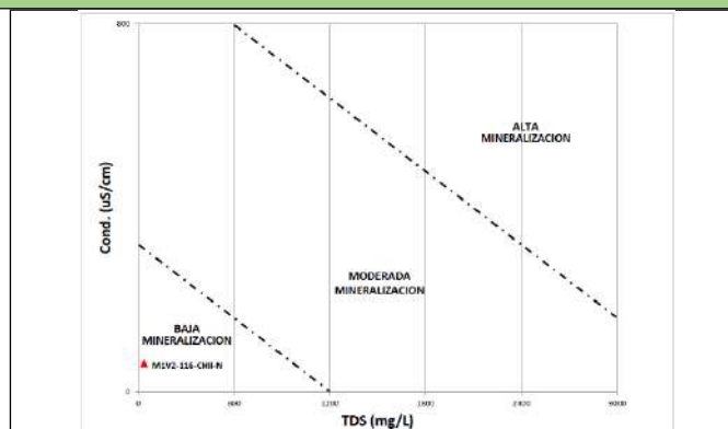
Diagrama TDS vs Conductividad muestra M1V2-116-CHII-N
