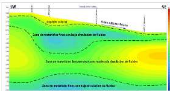
Figura 12. Modelo de resistividades construido con los sondeos 89-1, 68-1, 67-3 y 87-1
