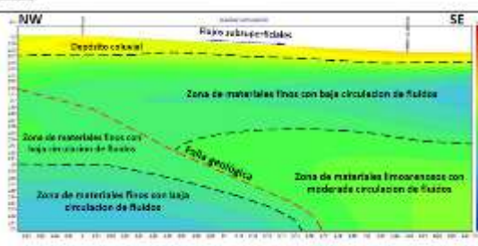
Figura 15. Modelo de resistividades construido con los sondeos 68-1 y 68-2
