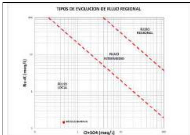
Diagrama evolución flujo muestra M1V2-116-CHII-N
