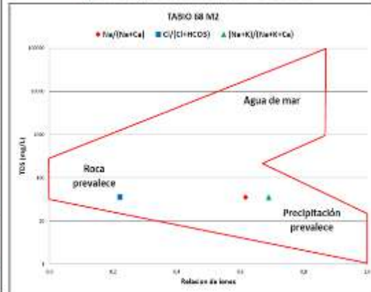
Figura 7-2. Diagrama de Gibbs muestra TABIO 68 M2
