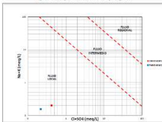
Figura 7-4. Diagrama Evolución de Flujo Regional
