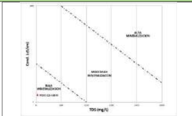
Diagrama TDS vs Conductividad muestra M1V2-116-CHII-N
