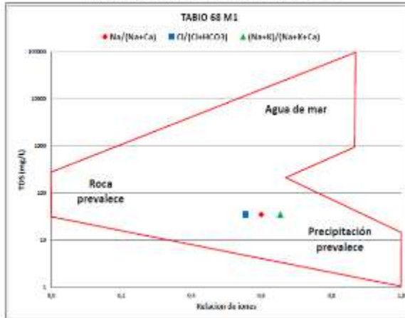
Figura 7-1. Diagrama de Gibbs muestra TABIO 68 M1
