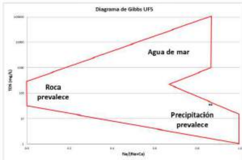
Figura 7-1. Diagrama de Gibbs
