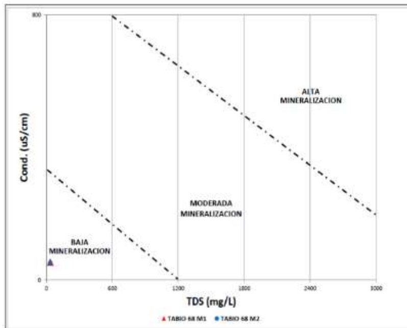
Figura 7-3. Diagrama de TDS vs Conductividad
