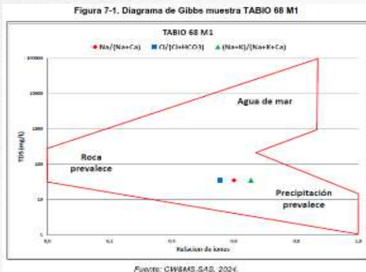
Diagrama de Gibbs muestras Tabio 68 M1 y Tabio 68 M2
