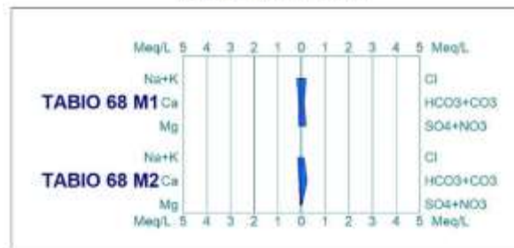
Figura 7-7. Diagrama Stiff
