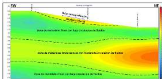
Figura 14. Modelo de resistividades construido con los sondeos 80-1, 67-015 y 67-1
