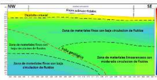
Figura 15. Modelo de resistividades construido con los sondeos 68-1 y 68-2
