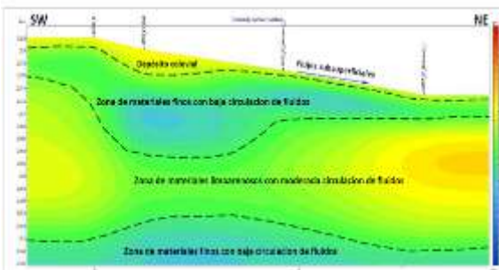
Figura 12. Modelo de resistividades construido con los sondeos 89-1, 68-1, 67-3 y 87-1
