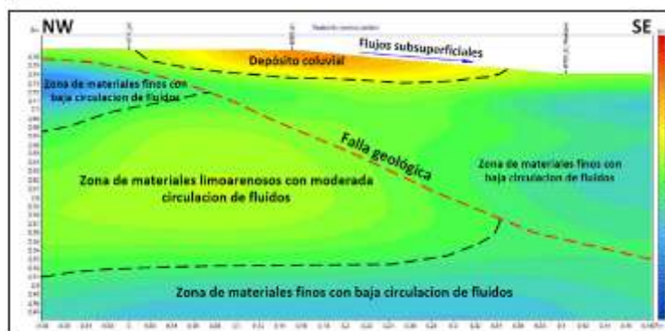
Figura 16. Modelo de resistividades construido con los sondeos 67-3, 67-1 y 67-2
