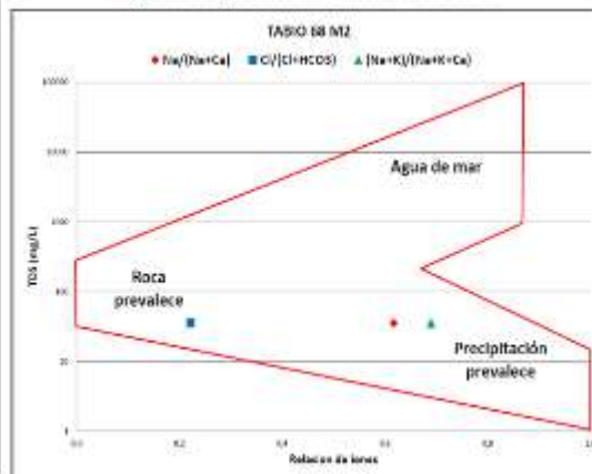
Figura 7-2. Diagrama de Gibbs muestra TABIO 68 M2
