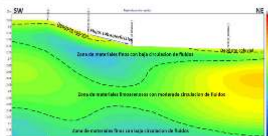
Figura 13. Modelo de resistividades construido con los sondeos 69-1, 68-2, 67-2 y 67-1
