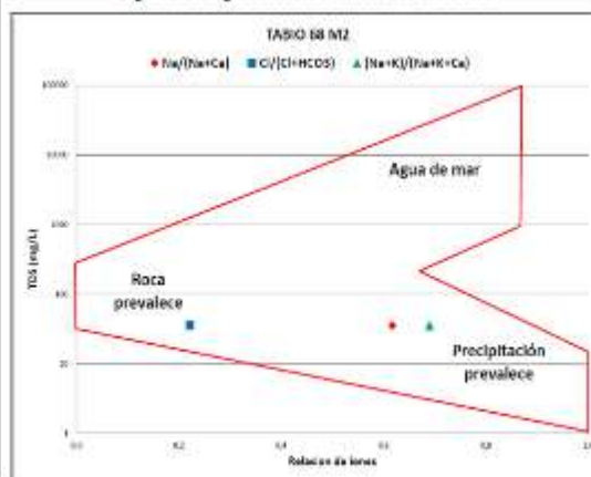
Figura 7-2. Diagrama de Gibbs muestra TABIO 68 M2
