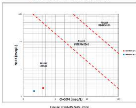
Figura 7-4. Diagrama Evolución de Flujo Regional
