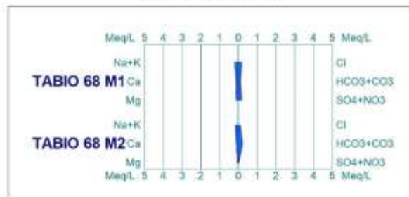
Figura 7-7. Diagrama Stiff
