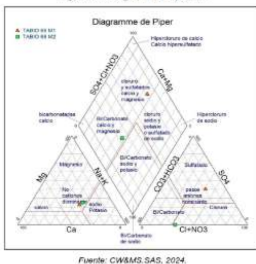
Figura 7-5. Diagrama de Piper Hill
