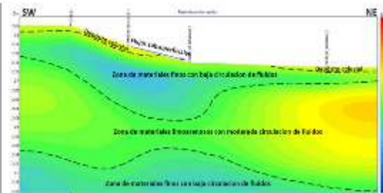
Figura 13. Modelo de resistividades construido con los sondeos 69-1, 68-2, 67-2 y 67-1
