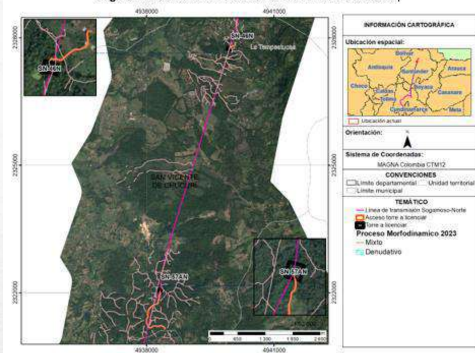
Figura 5-19 Procesos morfodinámicos sitios de torre|
